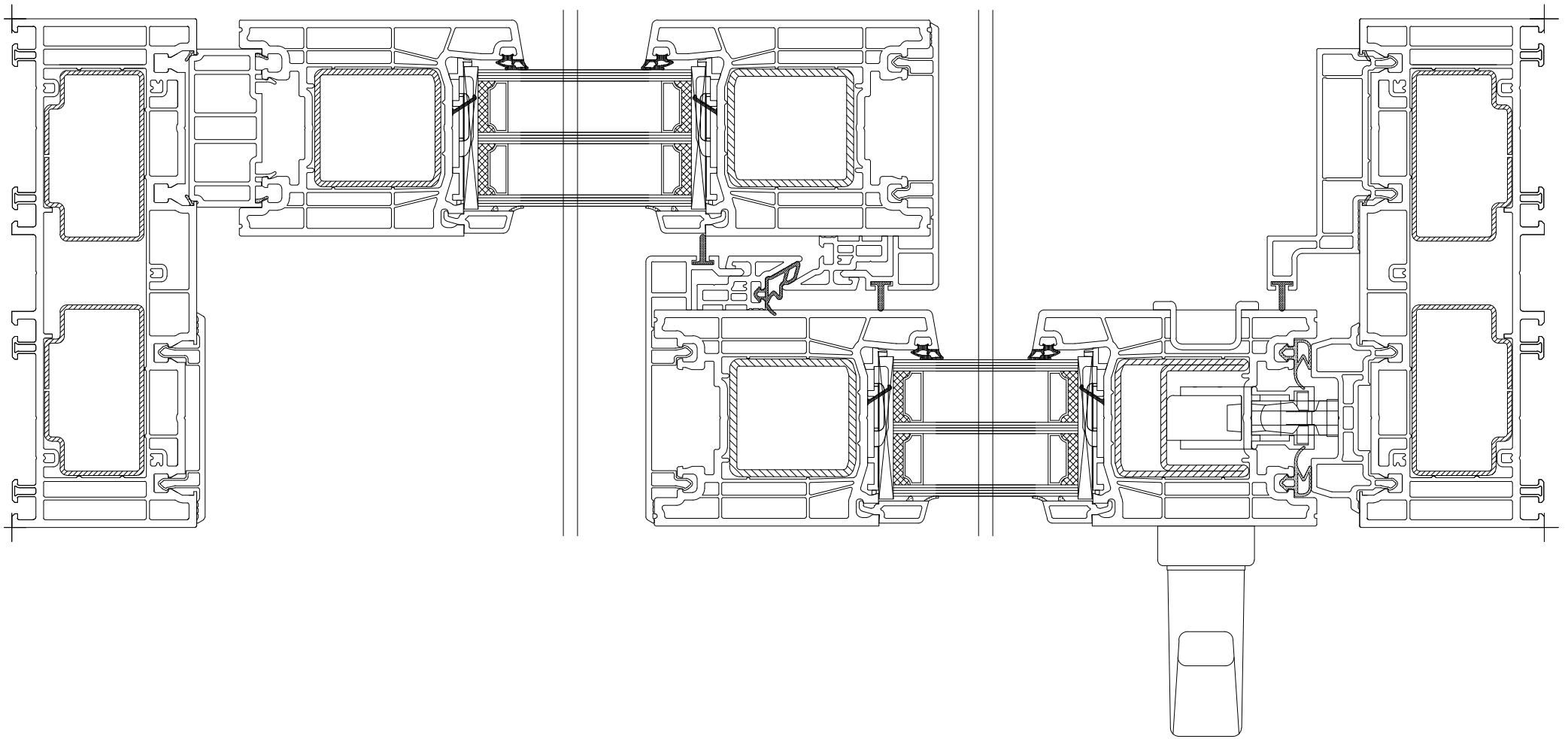
Coupe horizontale Porte-fenêtre à levage PremiDoor 76
